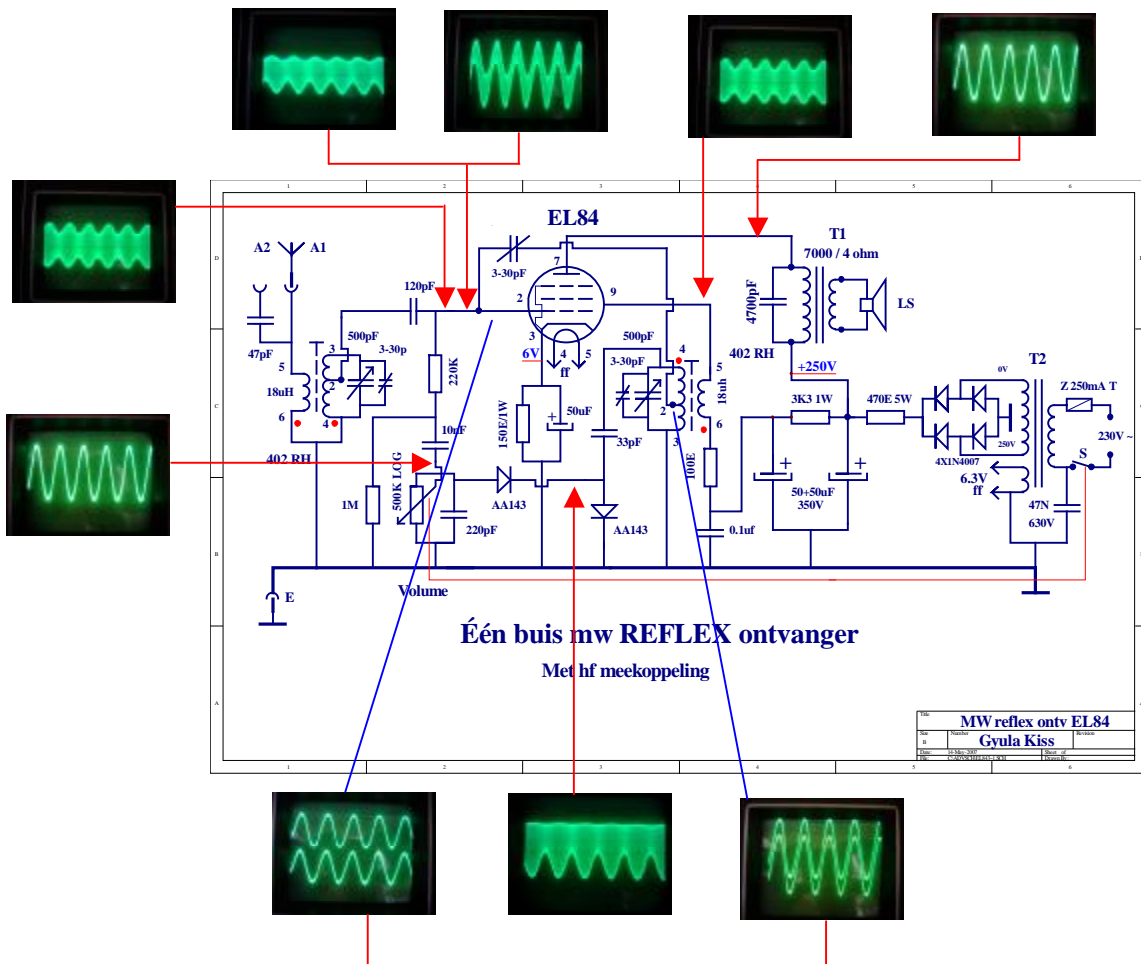
ÉÉNBUIS MW REFLEX ONTVANGER MET EL84 1+1 + hf meekoppeling
